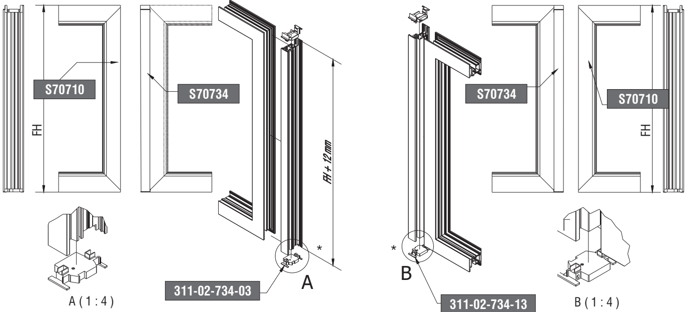
Χαμηλό κατωκάσι S70720 S70762 Low threshold S70720 S70762
