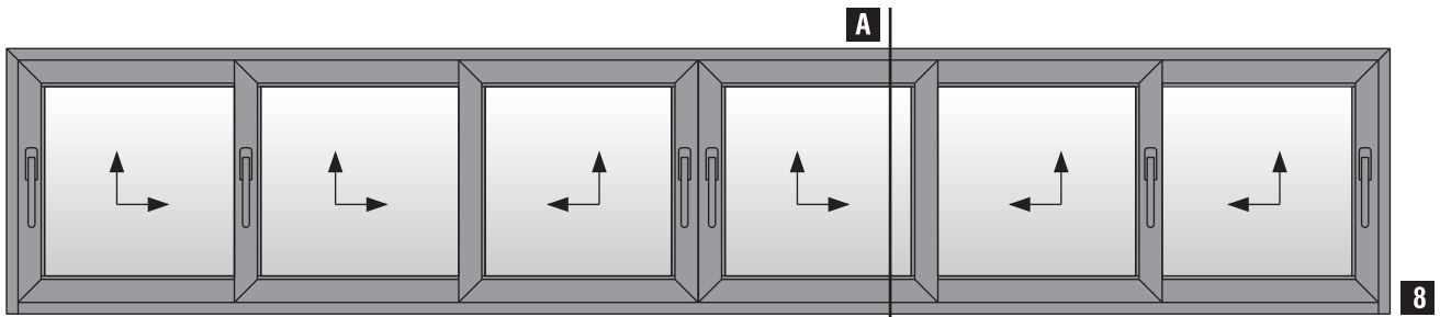
Εξάφυλλο επάλληλο φιλητό ανασυρόμενο με χρήση τριπλού οδηγού & χαμηλού οδηγού S70762 Six sash parallel meeting stile lift & slide with triple frame guide & S70762 short frame guide use
