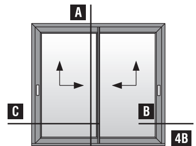
Δίφυλλο επάλληλο ανασυρόμενο ΑΡΙΣΤΕΡΟ με χρήση χαμηλού οδηγού S70720 Two sash parallel lift & slide LEFT with S70720 short frame guide use
