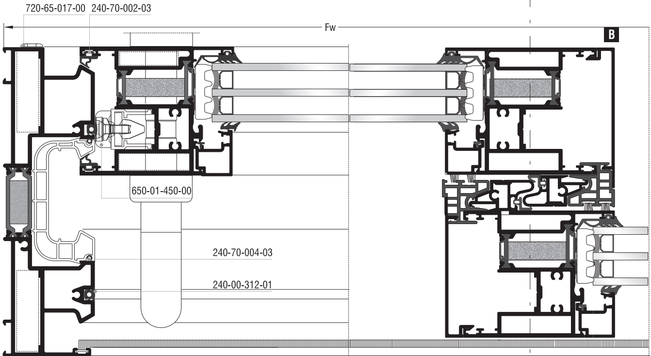
5B Τετράφυλλο φιλιτό επάλληλο ανασυρόμενο με χρήση χαμηλού οδηγού S70720 | Four sash parallel meeting stilet lift & slide with S70720 short frame guide use
