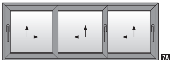
Τρίφυλλο επάλληλο ανασυρόμενο ΔΕΞΙ με χρήση χαμηλού οδηγού Three sash parallel lift & slide RIGHT with short frame guide use
