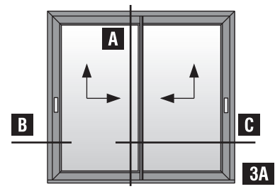
Δίφυλλο επάλληλο ανασυρόμενο ΔΕΞΙ με χρήση χαμηλού οδηγού S70720 (κοπή 90°) Two sash parallel lift & slide RIGHT with S70720 short frame guide use (90° cutting)
