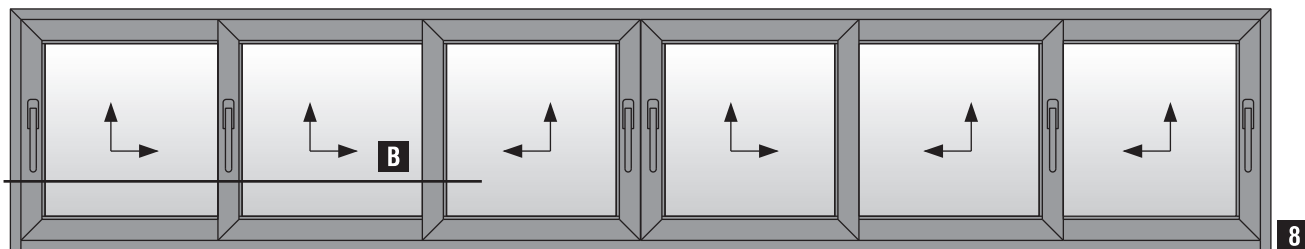
Εξάφυλλο επάλληλο φιλητό ανασυρόμενο με χρήση τριπλού οδηγού & χαμηλού οδηγού S70762 Six sash parallel meeting stile lift & slide with triple frame guide & S70762 short frame guide use
