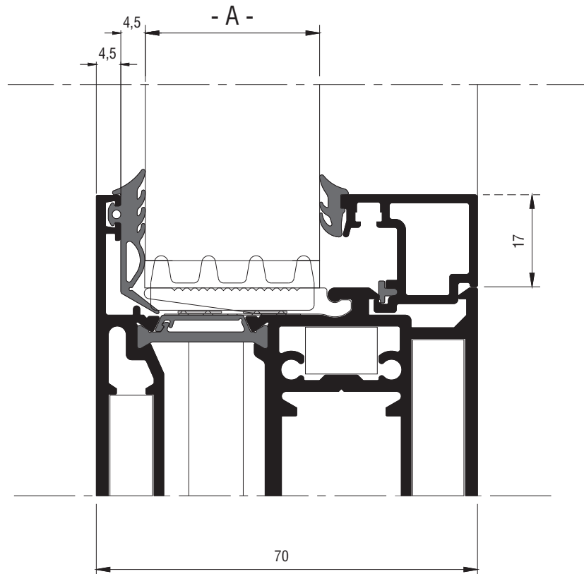
Ενδεικτική τομή - Indicative section
