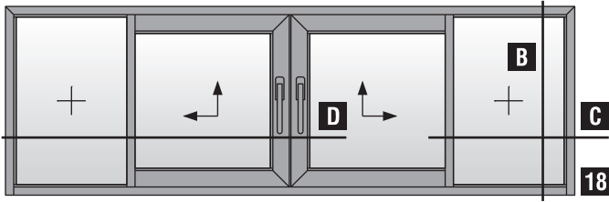
Δίφυλλο φιλιτό αριστερά ανασυρόμενο με σταθερά Two sash meeting stile left lift & slide with fixed
