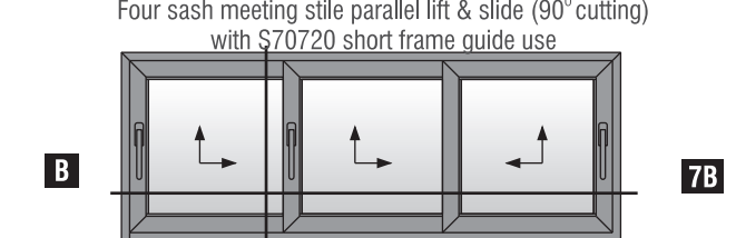
Τρίφυλλο επάλληλο ανασυρόμενο ΑΡΙΣΤΕΡΟ με χρήση χαμηλού οδηγού Three sash parallel lift & slide LEFT with short frame guide use
