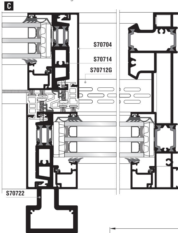
Δίφυλλο φιλιτό αριστερά ανασυρόμενο με σταθερά Two sash meeting stile left lift & slide with fixed
