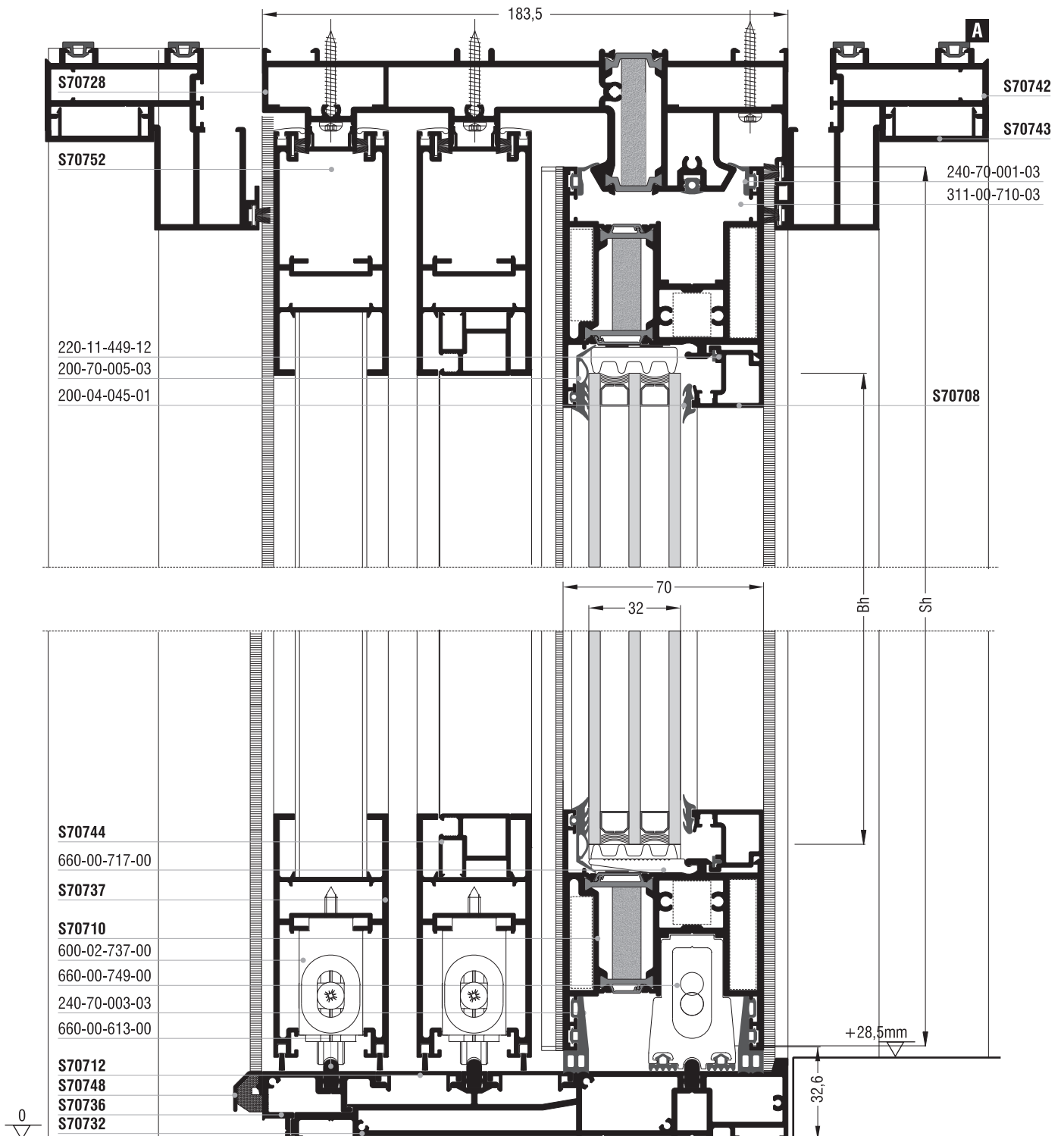
Δίφυλλο φιλητό χωνευτό ανασυρόμενο παράθυρο με σήτα και παντζούρι Two sash meeting stile pocket & slide window with fly-screen and shutter
