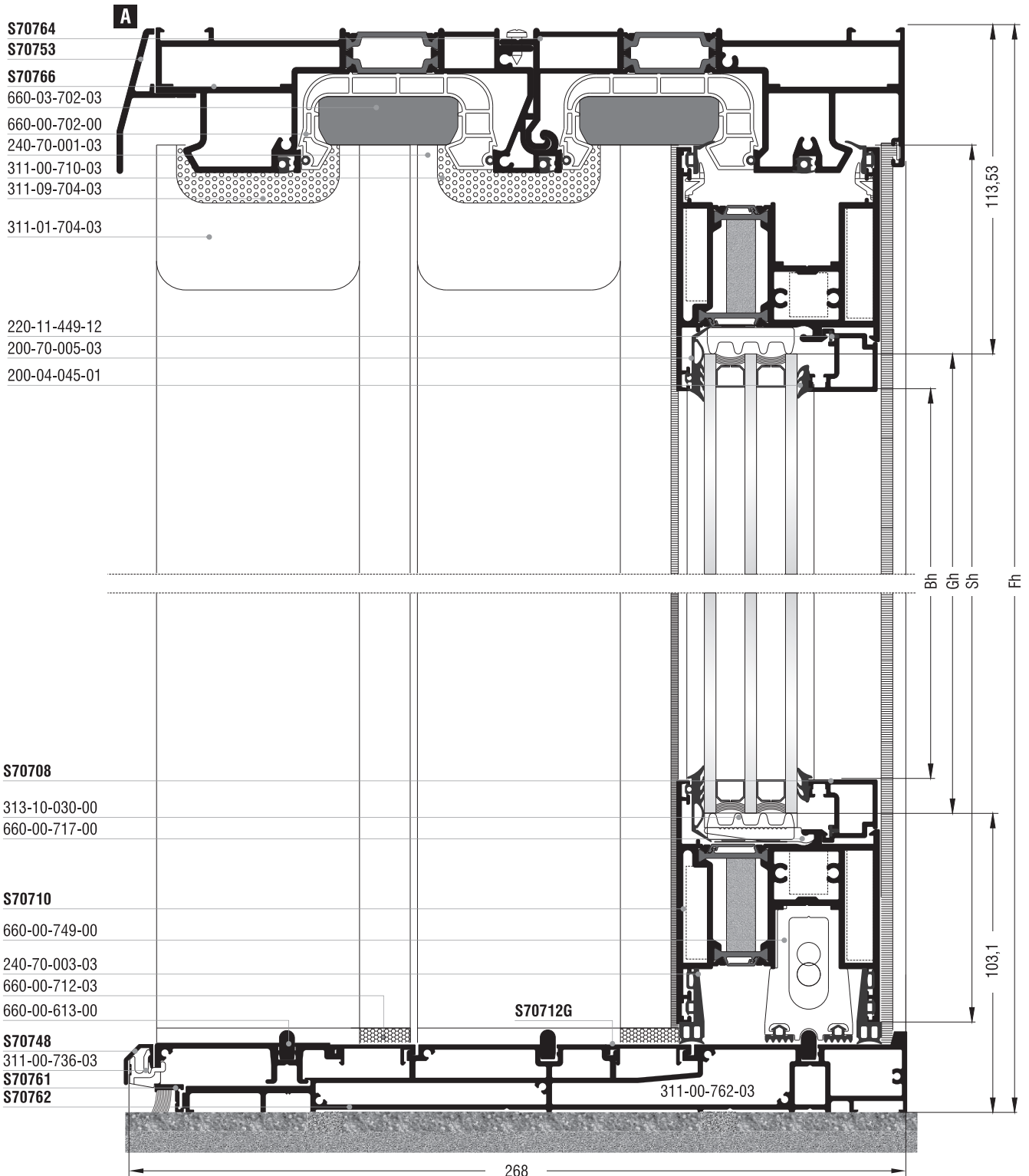
Εξάφυλλο επάλληλο φιλητό ανασυρόμενο με χρήση τριπλού οδηγού & χαμηλού οδηγού S70762 Six sash parallel meeting stile lift & slide with triple frame guide & S70762 short frame guide use
