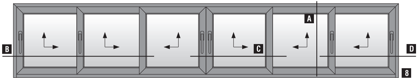
Εξάφυλλο επάλληλο φιλητό ανασυρόμενο με χρήση τριπλού οδηγού & χαμηλού οδηγού S70762 Six sash parallel meeting stile lift & slide with triple frame guide & S70762 short frame guide use
