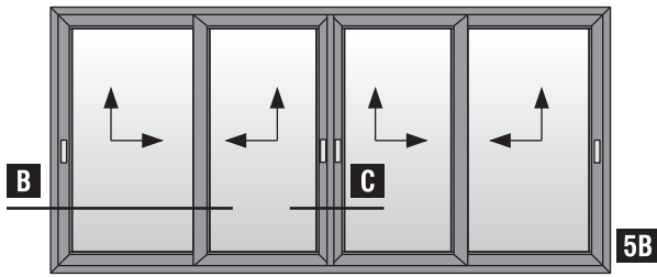
5B Τετράφυλλο φιλιτό επάλληλο ανασυρόμενο με χρήση χαμηλού οδηγού S70720 | Four sash parallel meeting stilet lift & slide with S70720 short frame guide use
