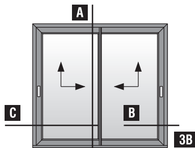
Δίφυλλο επάλληλο ανασυρόμενο ΑΡΙΣΤΕΡΟ με χρήση χαμηλού οδηγού S70720 (κοπή 90°) Two sash parallel lift & slide LEFT with S70720 short frame guide use (90° cutting)
