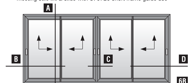
Τετράφυλλο φιλιτό επάλληλο ανασυρόμενο (κοπή 90°) με χρήση χαμηλού οδηγού S70720 Four sash meeting stile parallel lift & slide (90° cutting) with S70720 short frame guide use
