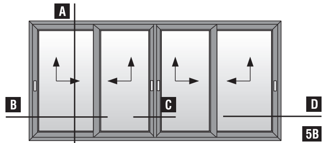
Τετράφυλλο φιλιτό επάλληλο ανασυρόμενο με χρήση χαμηλού οδηγού S70720 | Four sash parallel meeting stile lift & slide with S70720 short frame guide use
